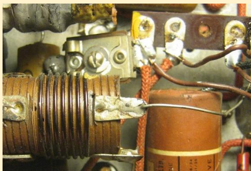
מעגלים אלקטרוניים מלפני כ-90 שנה, רכיבים מחוברים זה לזה באמצעות תגי הלחמה
